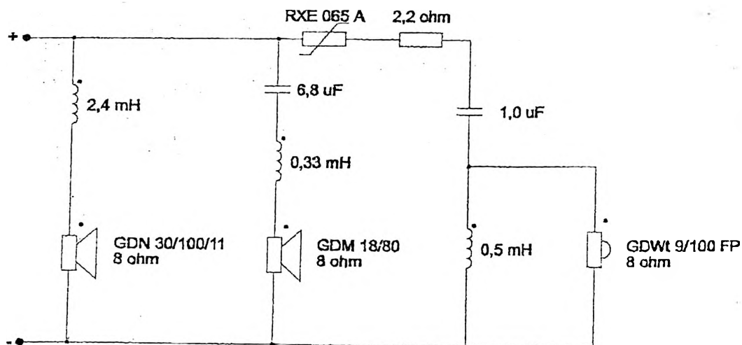
SCHEMAT ZWROTNICY ELEKTRYCZNEJ
