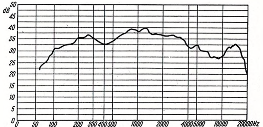
Rys. 5. Typowy przebieg charakterystyki przeniesienia zestawu głośnikowego typu ZG-8-114
