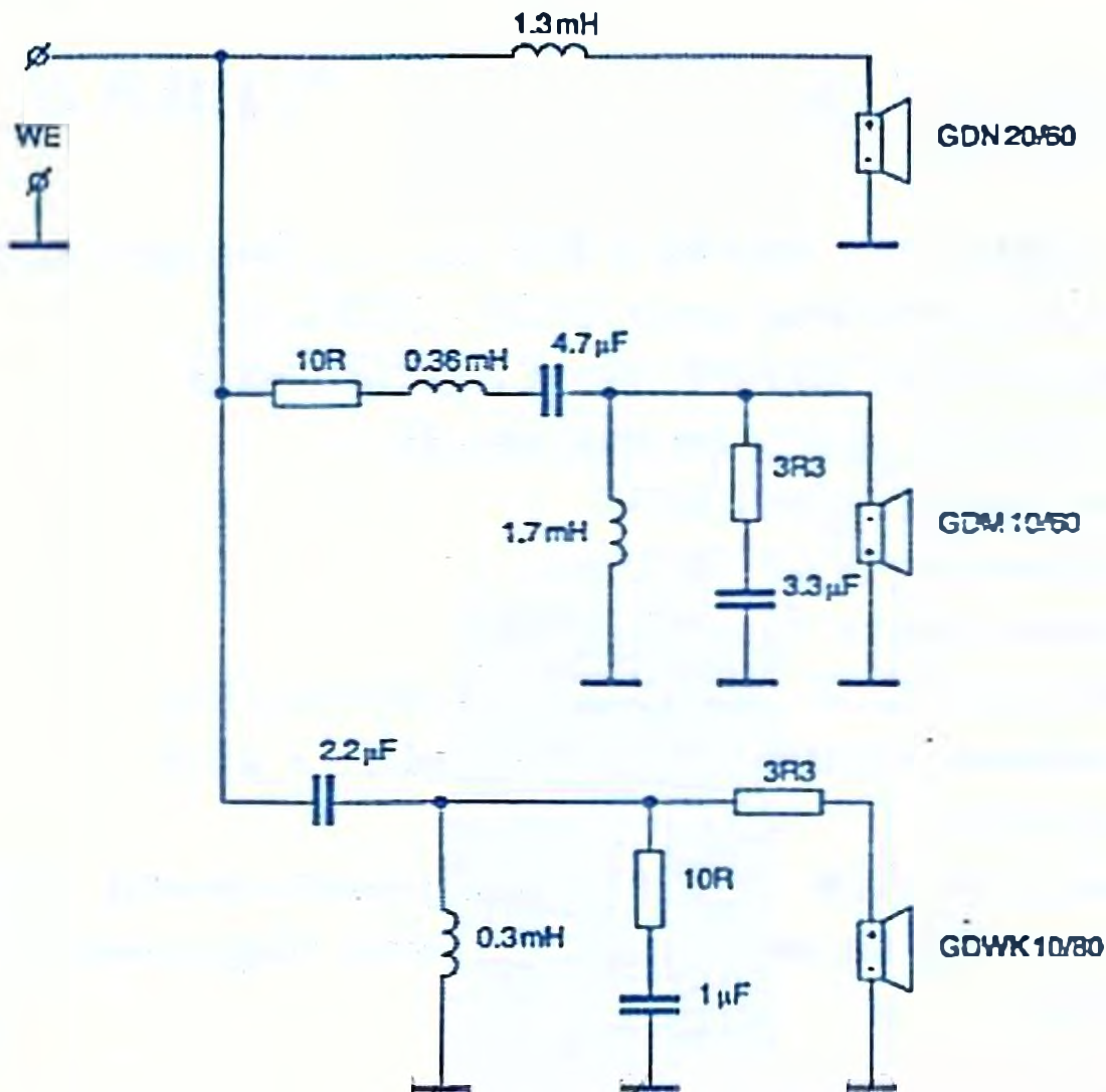
Schemat ideowy zestawu głośnikowego ZgB-80-8-903
