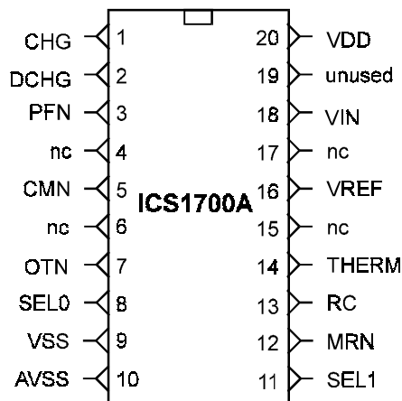
20-Pin SOIC
