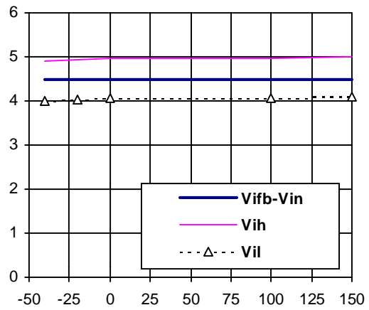
Figure 11 - Vih, Vil & Vfb-Vin (V) vs Tj (°C)
