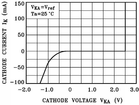
I_K - V_{KA}
