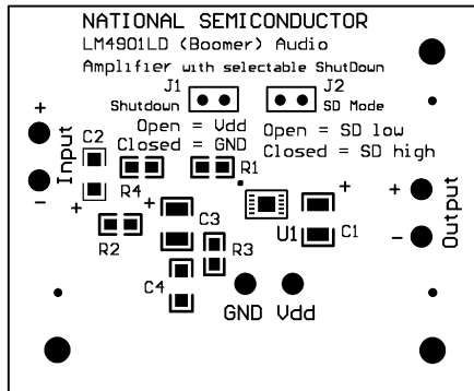
Figure 20. Top Layer
