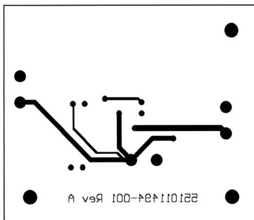
Figure 17. Bottom Layer
