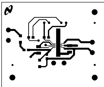
Figure 21. Bottom Layer
