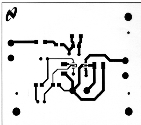
Figure 17. Bottom Layer
