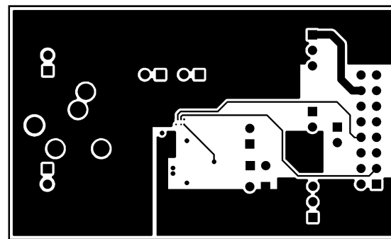
Figure 41. Bottom Layer
