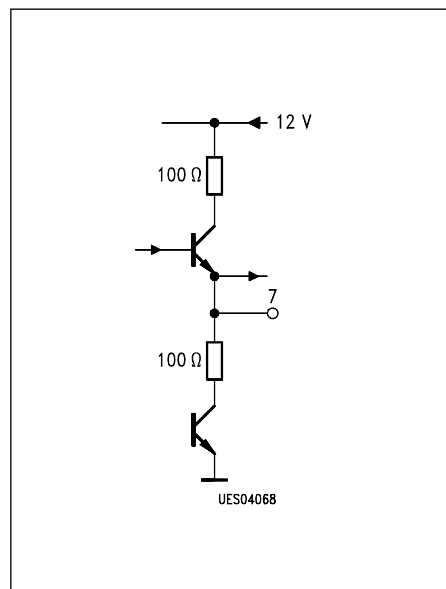
BASE2 (Pin 7)
