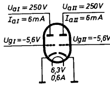
Meßschaltung
