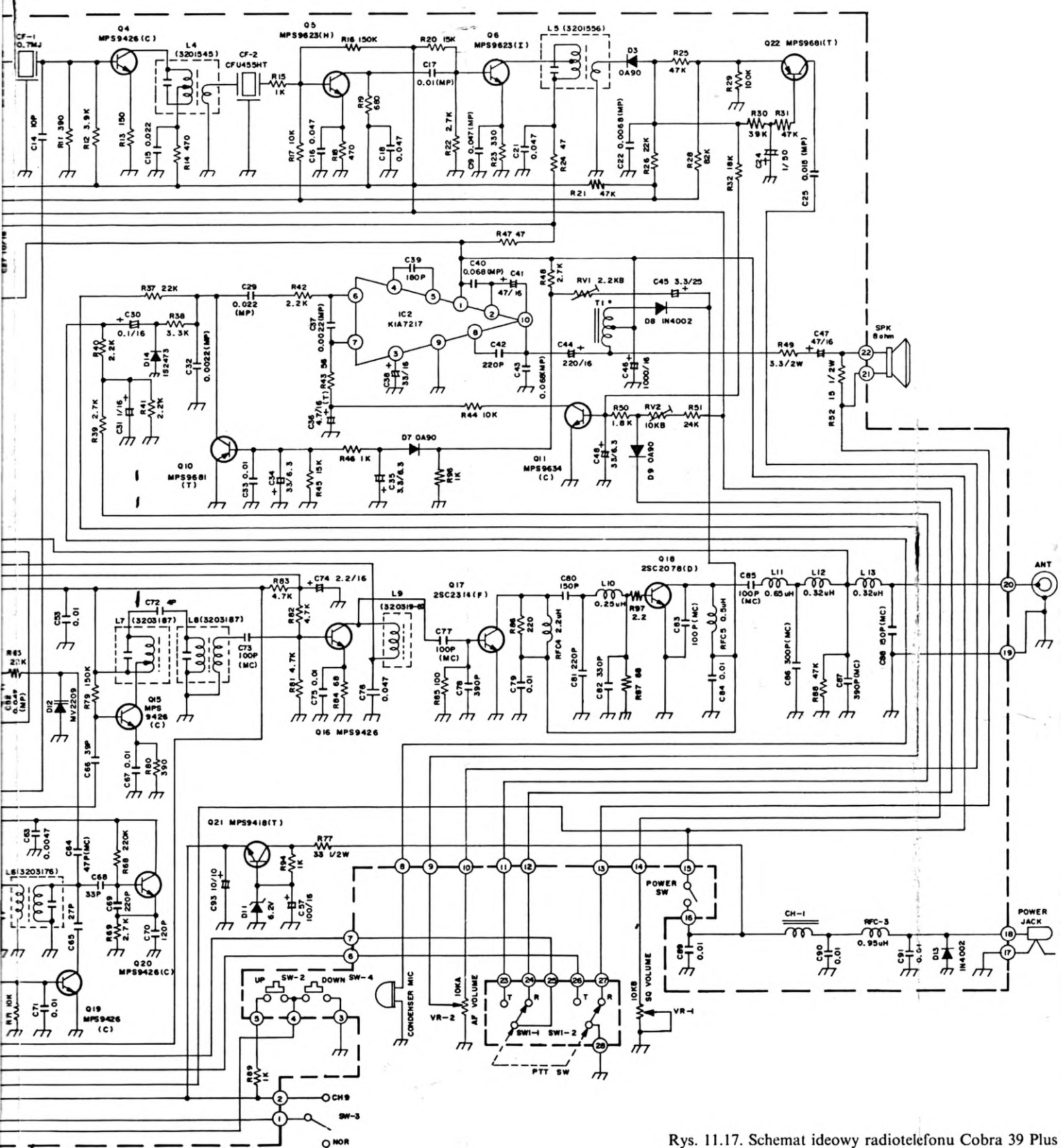
Rys. 11.17. Schemat ideowy radiotelefonu Cobra 39 Plus
