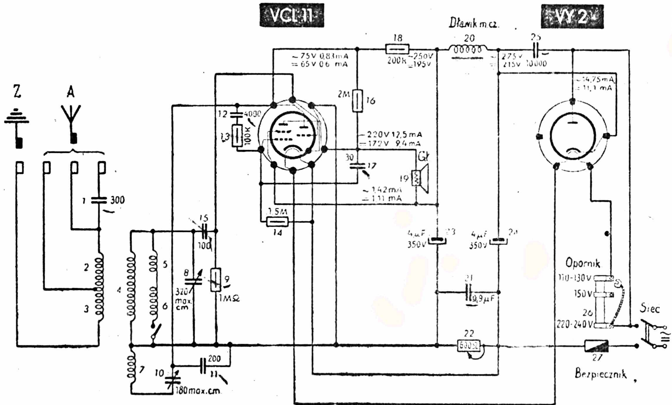
SCHEMAT RADIOODBIORNIKA TYPU „DKE 1938“.
