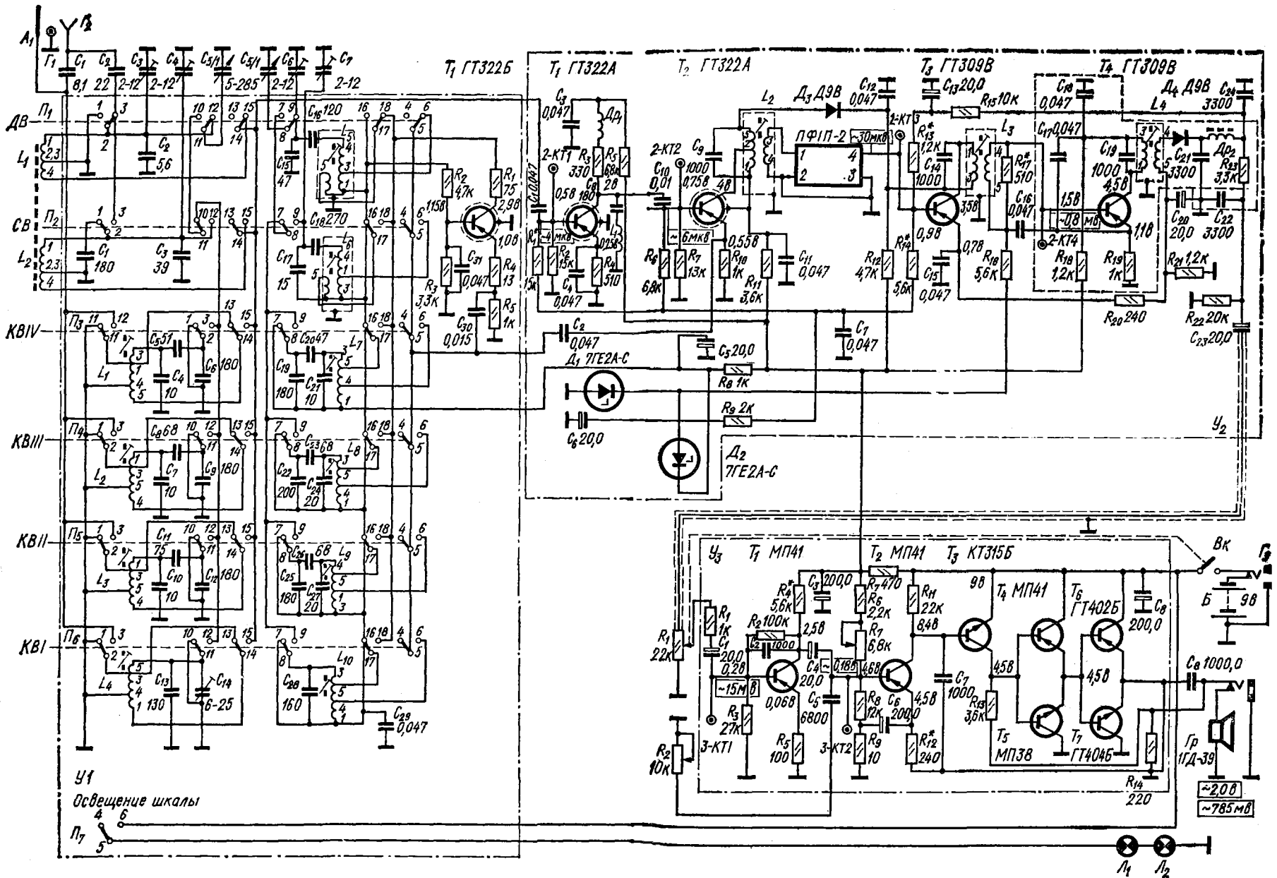
Принципиальная электрическая схема радиоприемника "Геолог" (переключатель диапазонов в положении ДВ).
