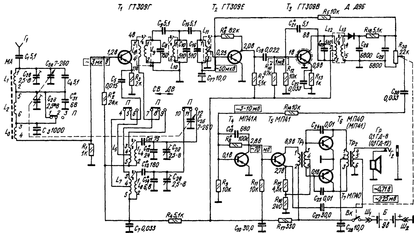
Принципиальная электрическая схема радиоприемников «Юпитер-601», «Юпитер-М»
