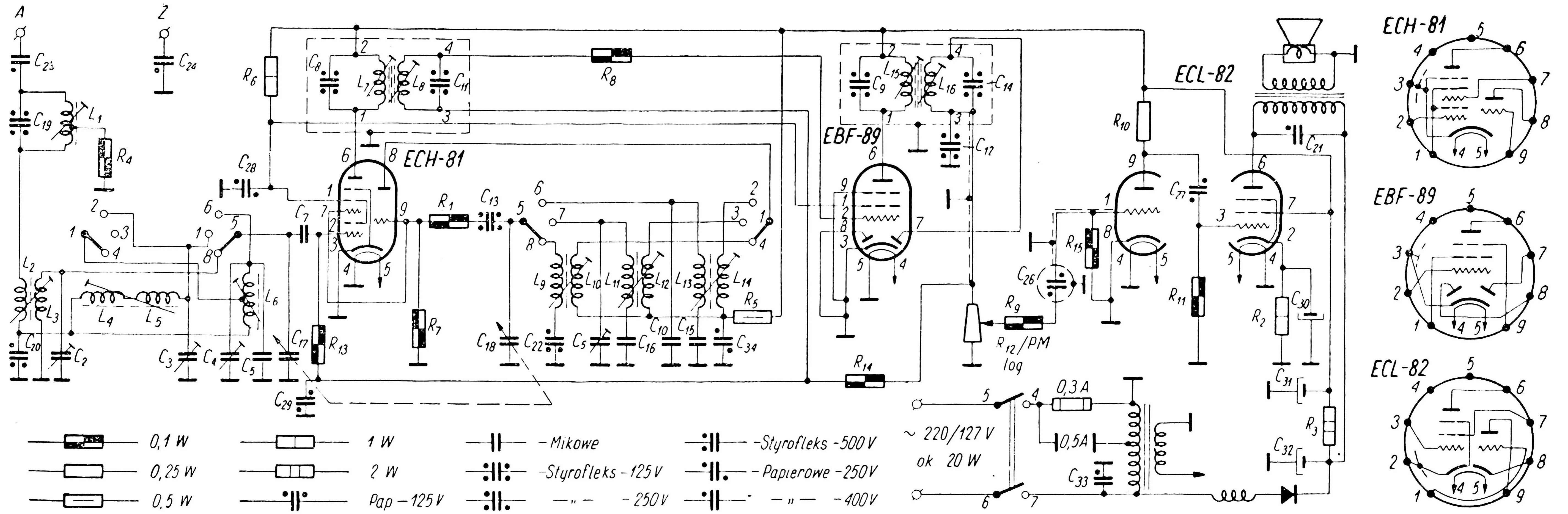
Schemat ideowy odbiornika „Kos“
