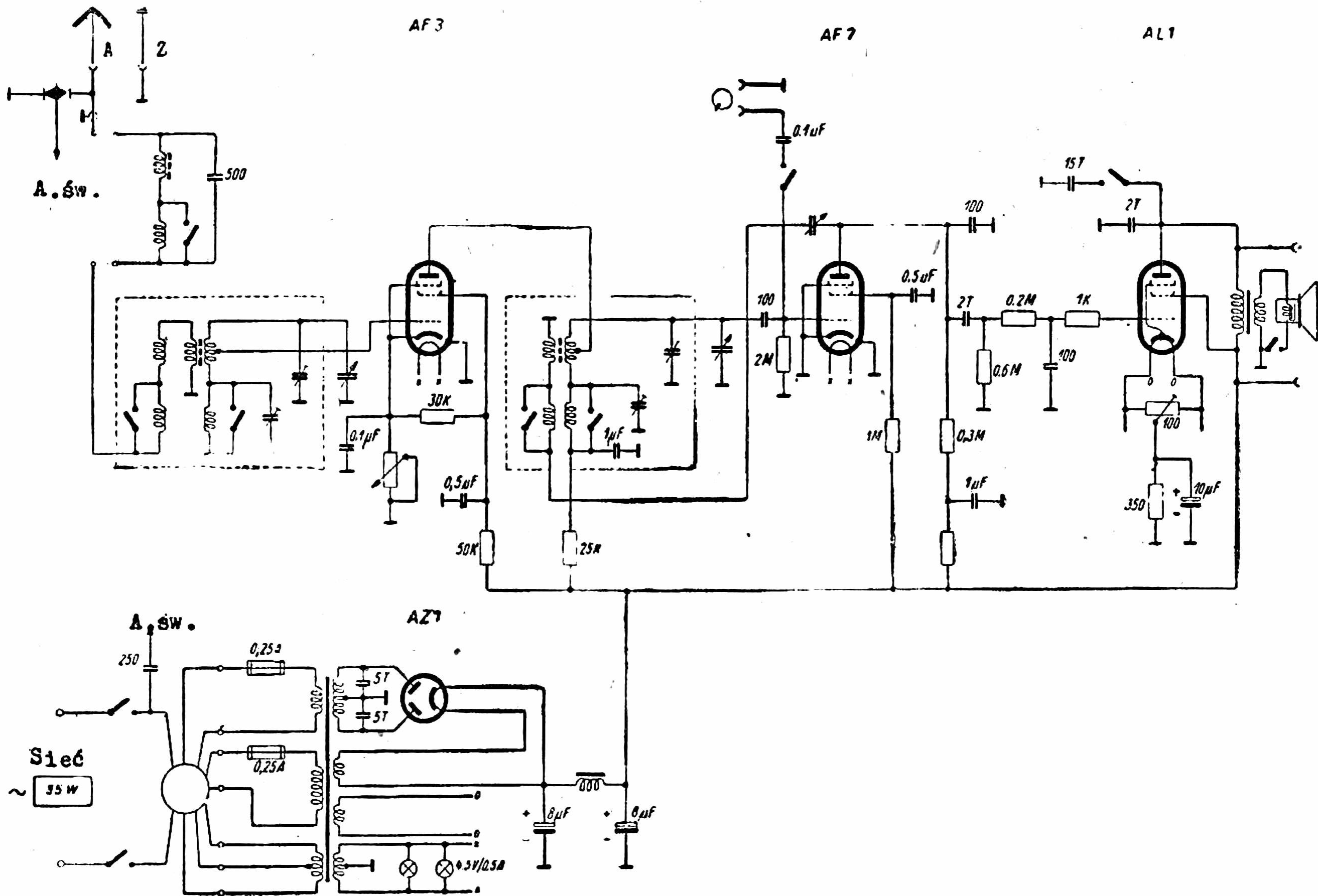
Schemat odbiornika Philips Aladin D23W
