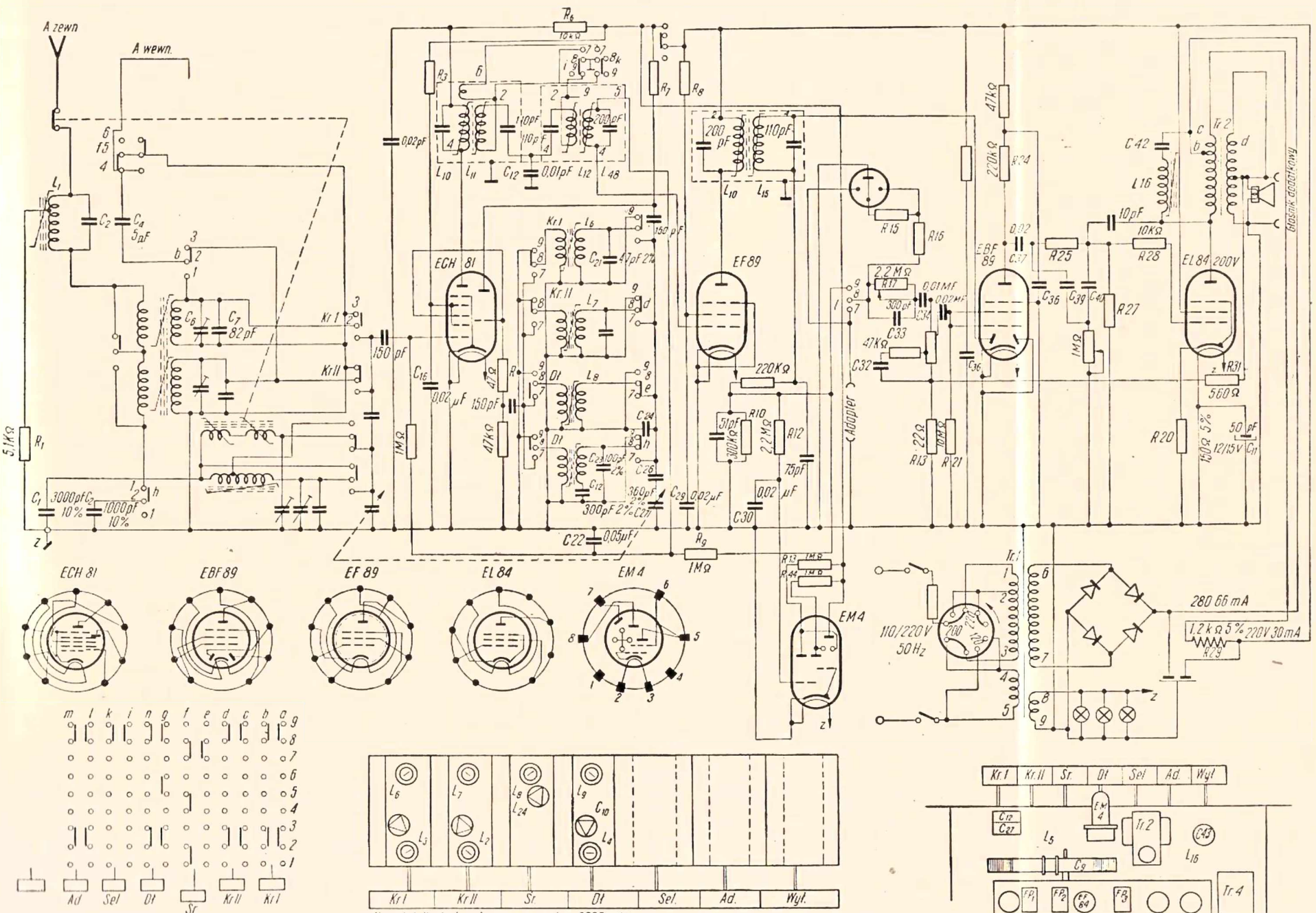
Rys. 21-10. Odbiornik „Rapsodia” z układem przemienny (trioda heksoda ECH81)
