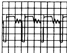
⑰ 440 Vp-p
